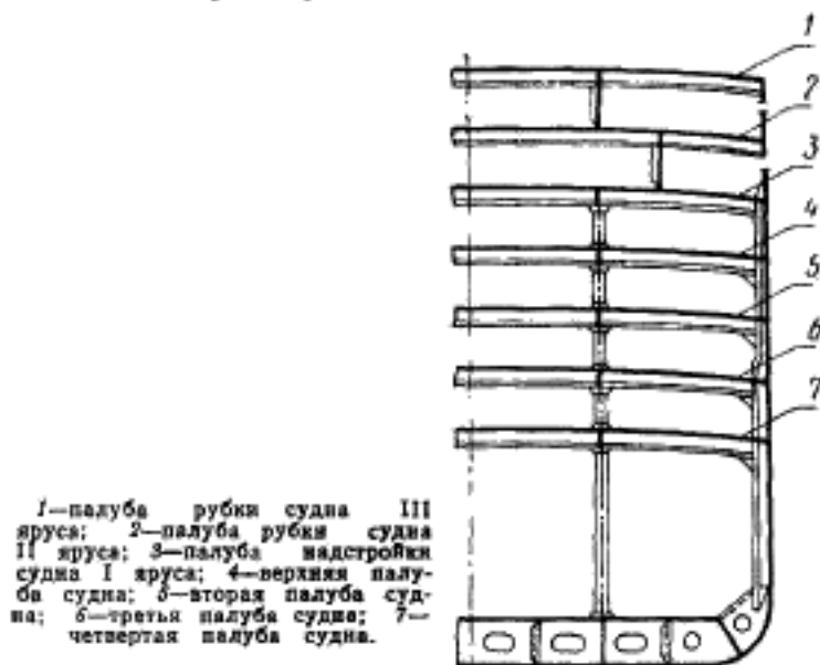
Черт. 1 Схема расположения палуб на судне
